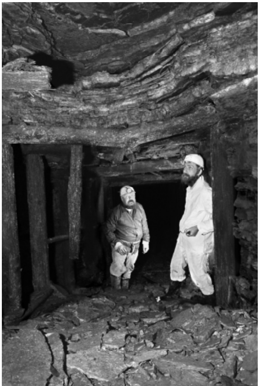
Rudník (v Podkrkonoší) – štola Jindřich, strop B (foto R. Tásler)
